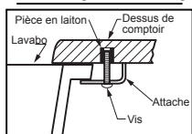
Détail de l'agrafe de montage
